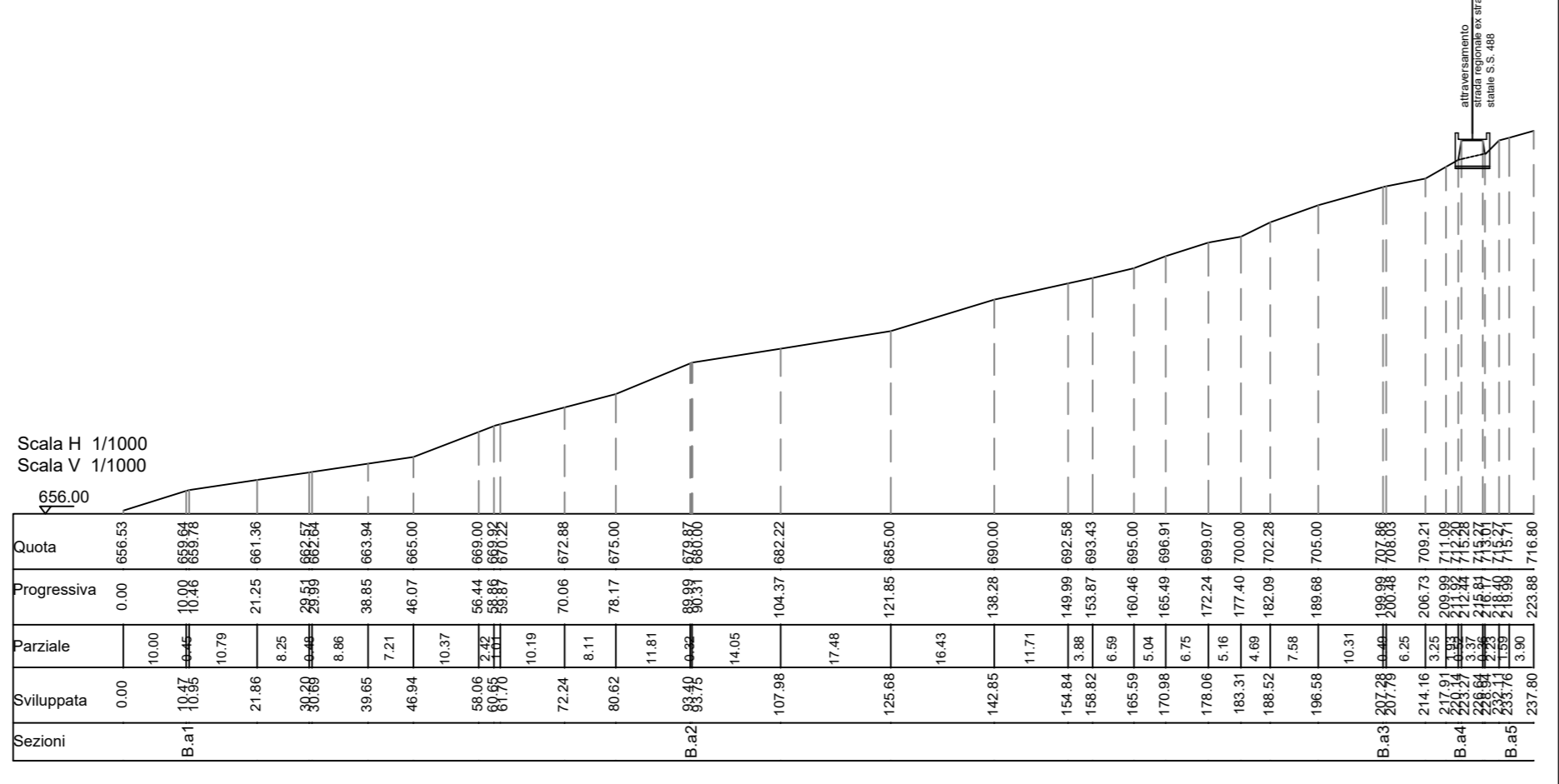
Profilo longitudinale asta "B.a"
