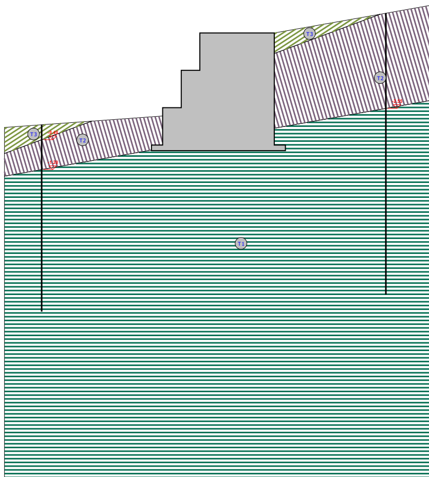
Vista Stratigrafica
