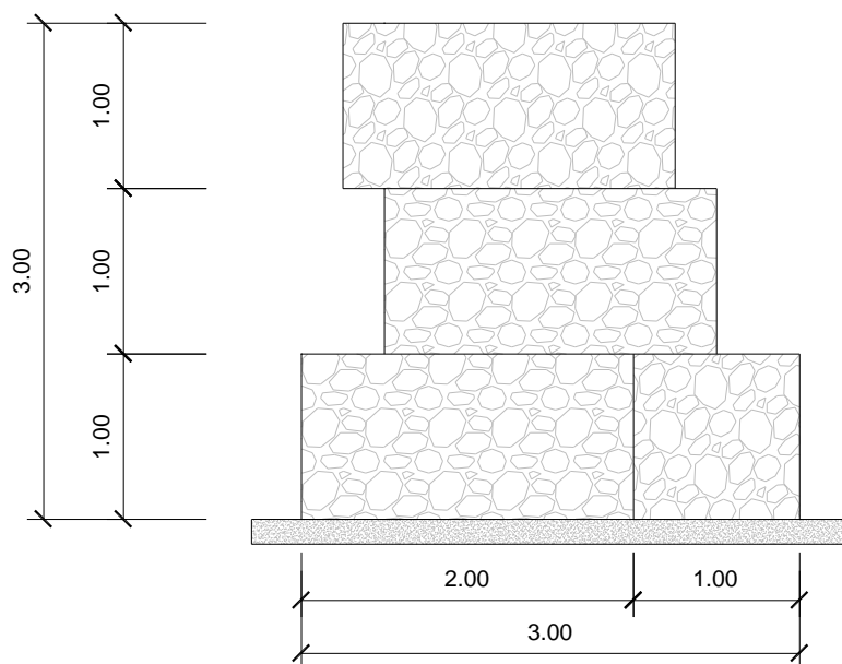
Vista Stratigrafica
