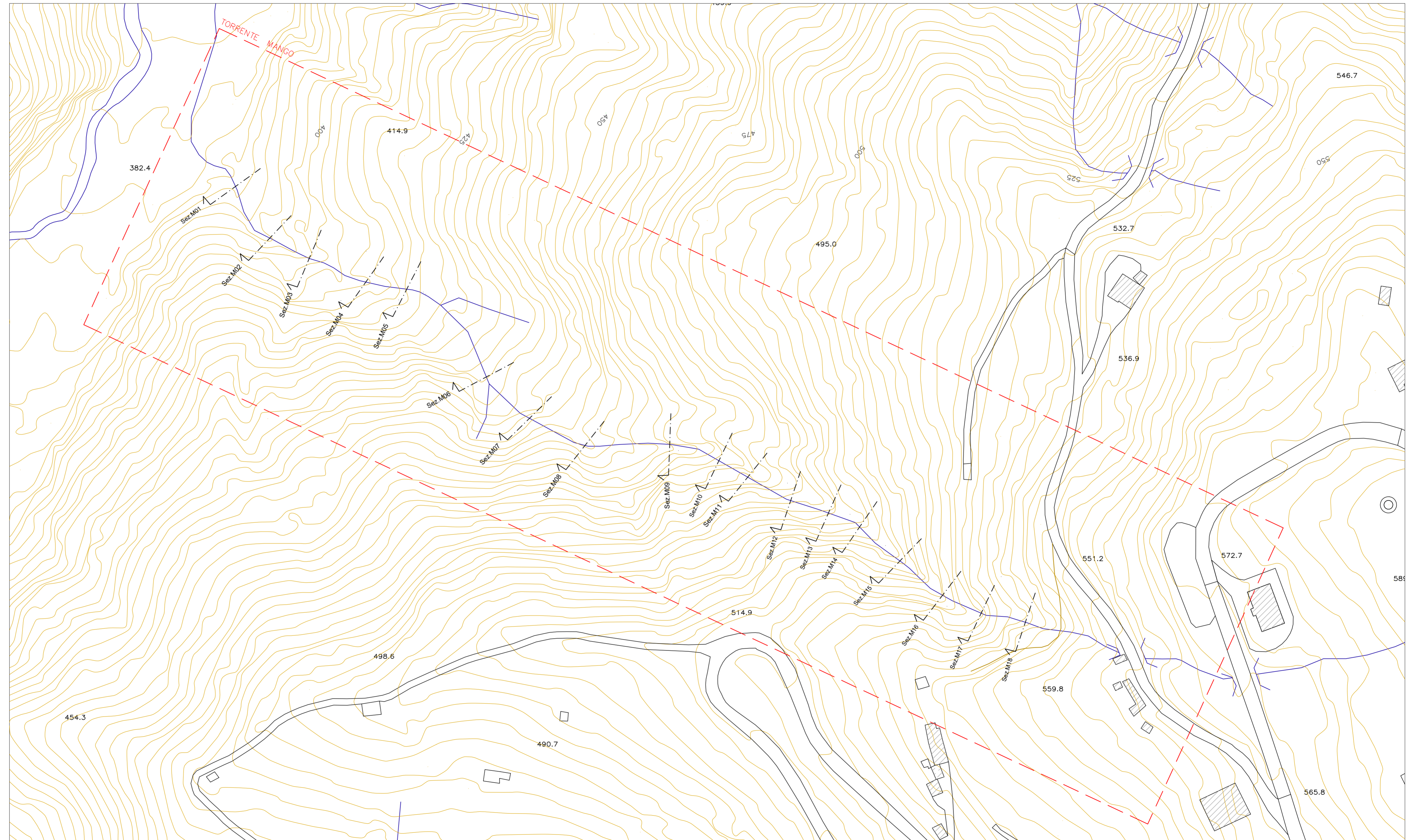
PLANIMETRIA STATO DI FATTO - TORRENTE MANGO scala 1:1000
