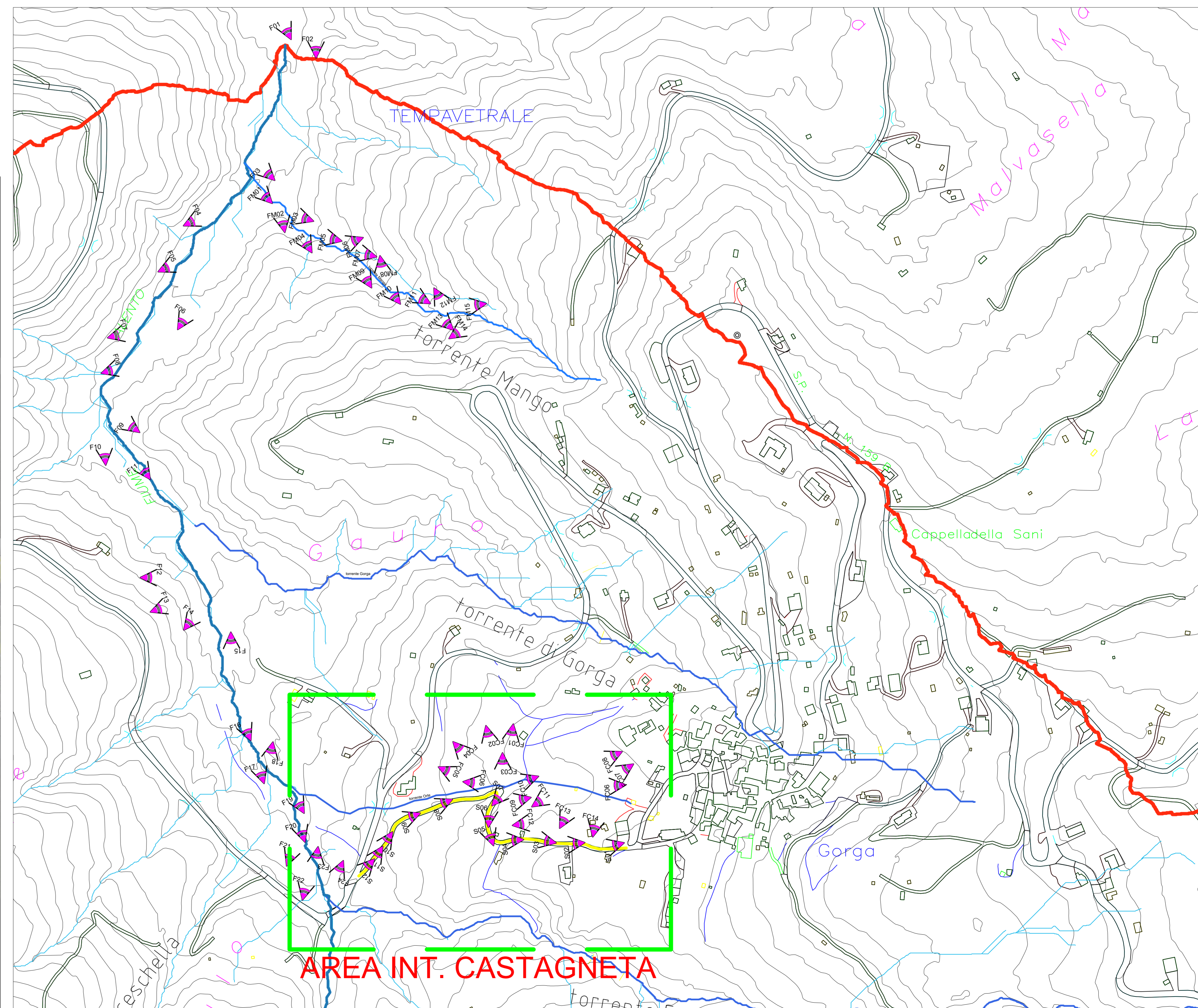
Planim. con punti di scatto
