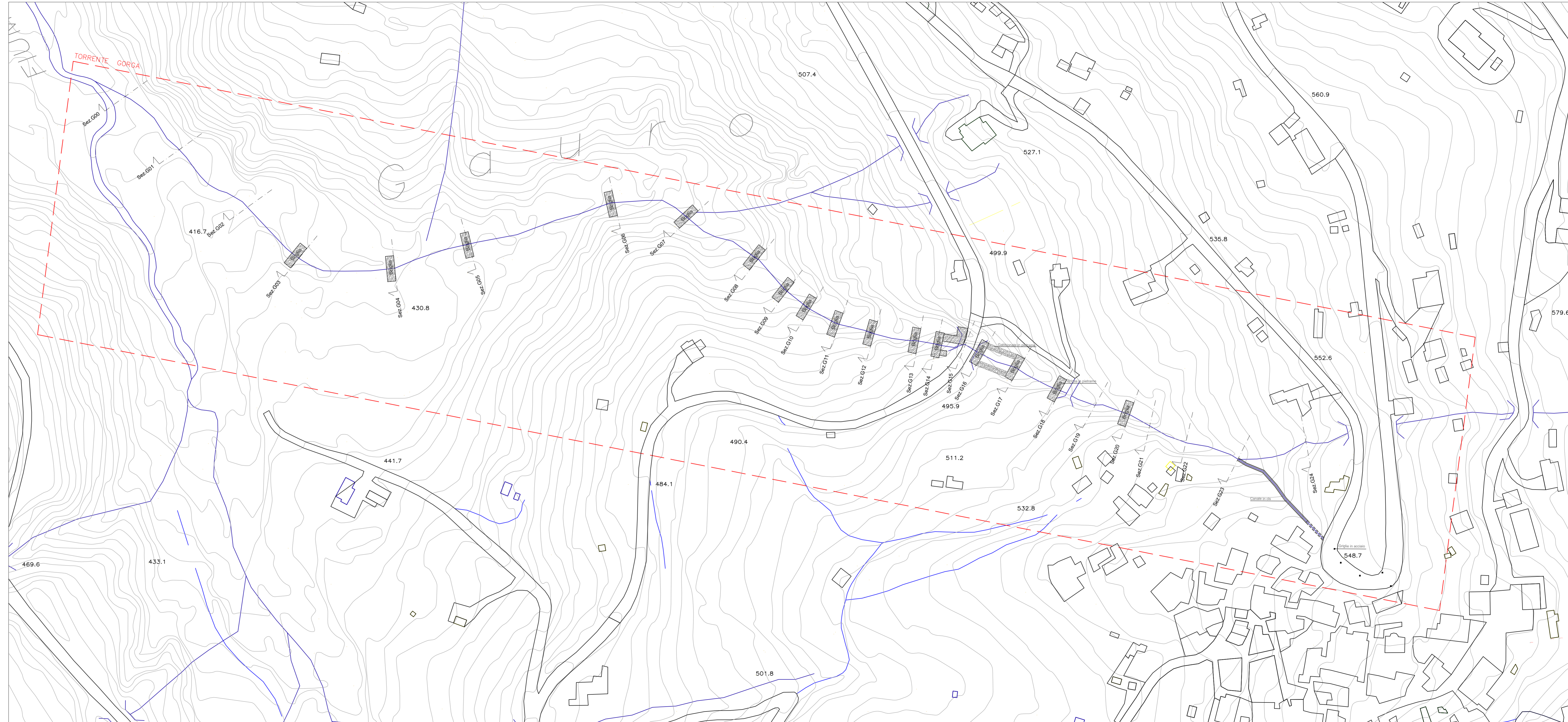
PLANIMETRIA STATO DI FATTO - TORRENTE GORGA scala 1:1000
