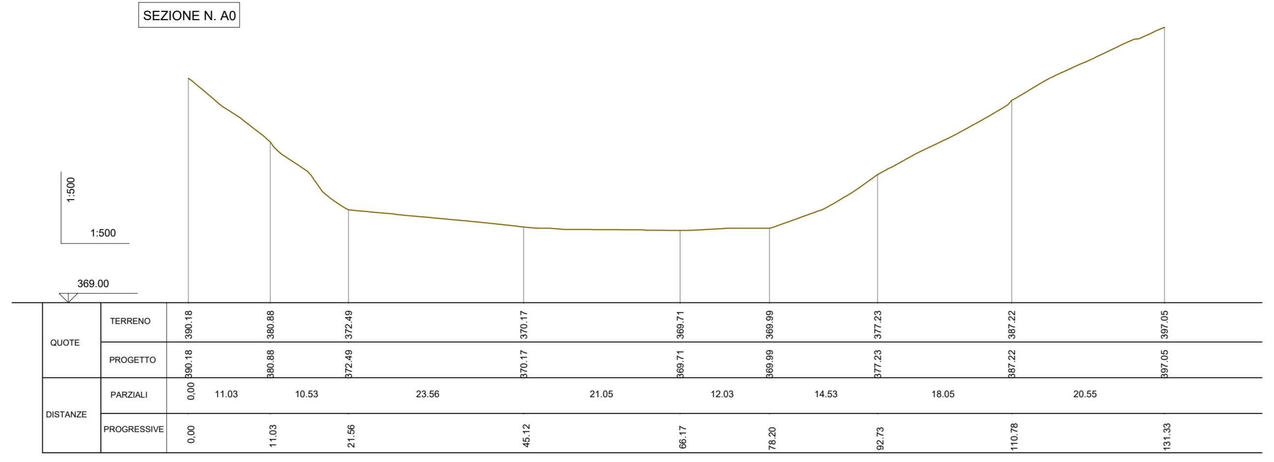
SEZIONI TRASVERSALI STATO DI PROGETTO scala 1:500
