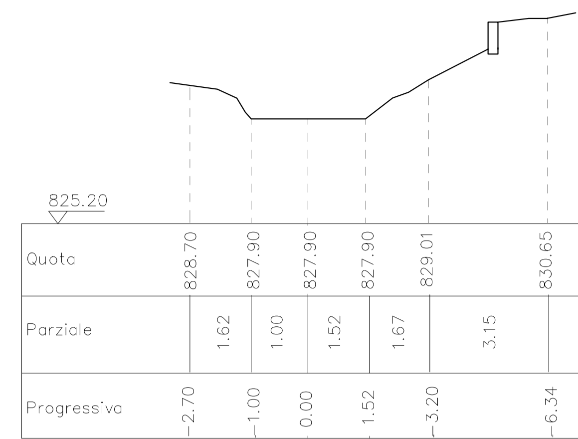
Stato di fatto sezione S3
