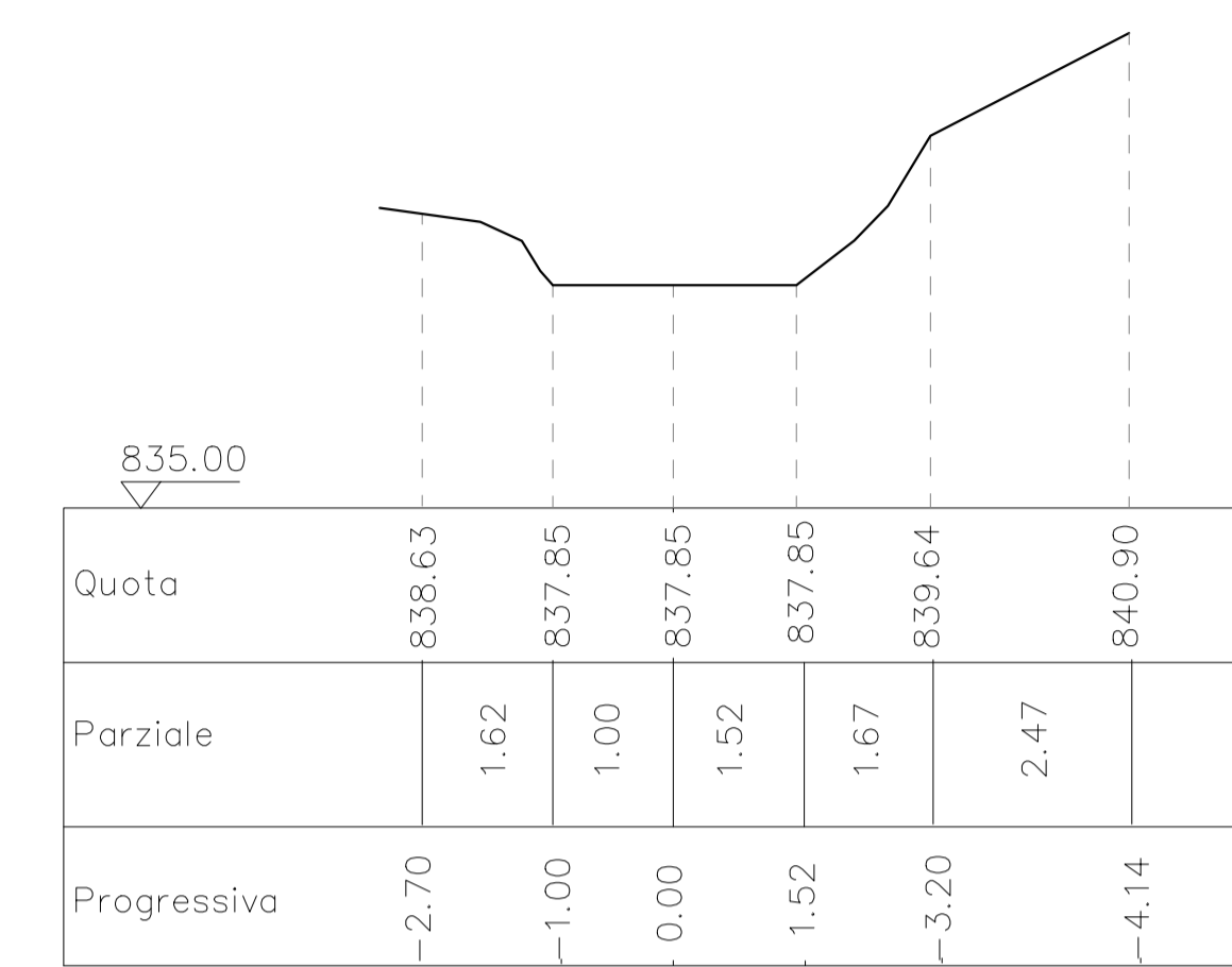
Stato di fatto sezione S5
