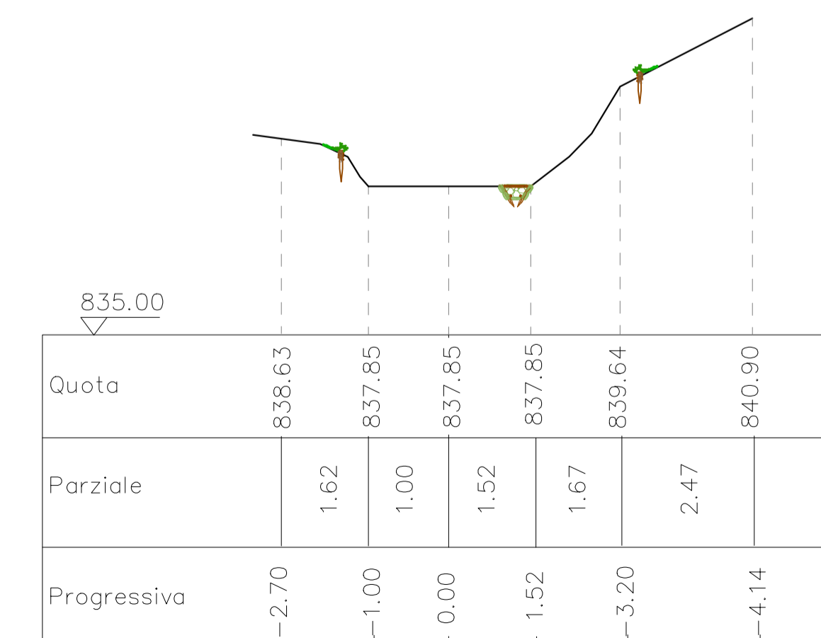
Progetto sezione S5
