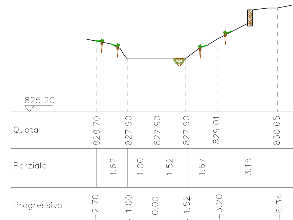
Progetto sezione S3
