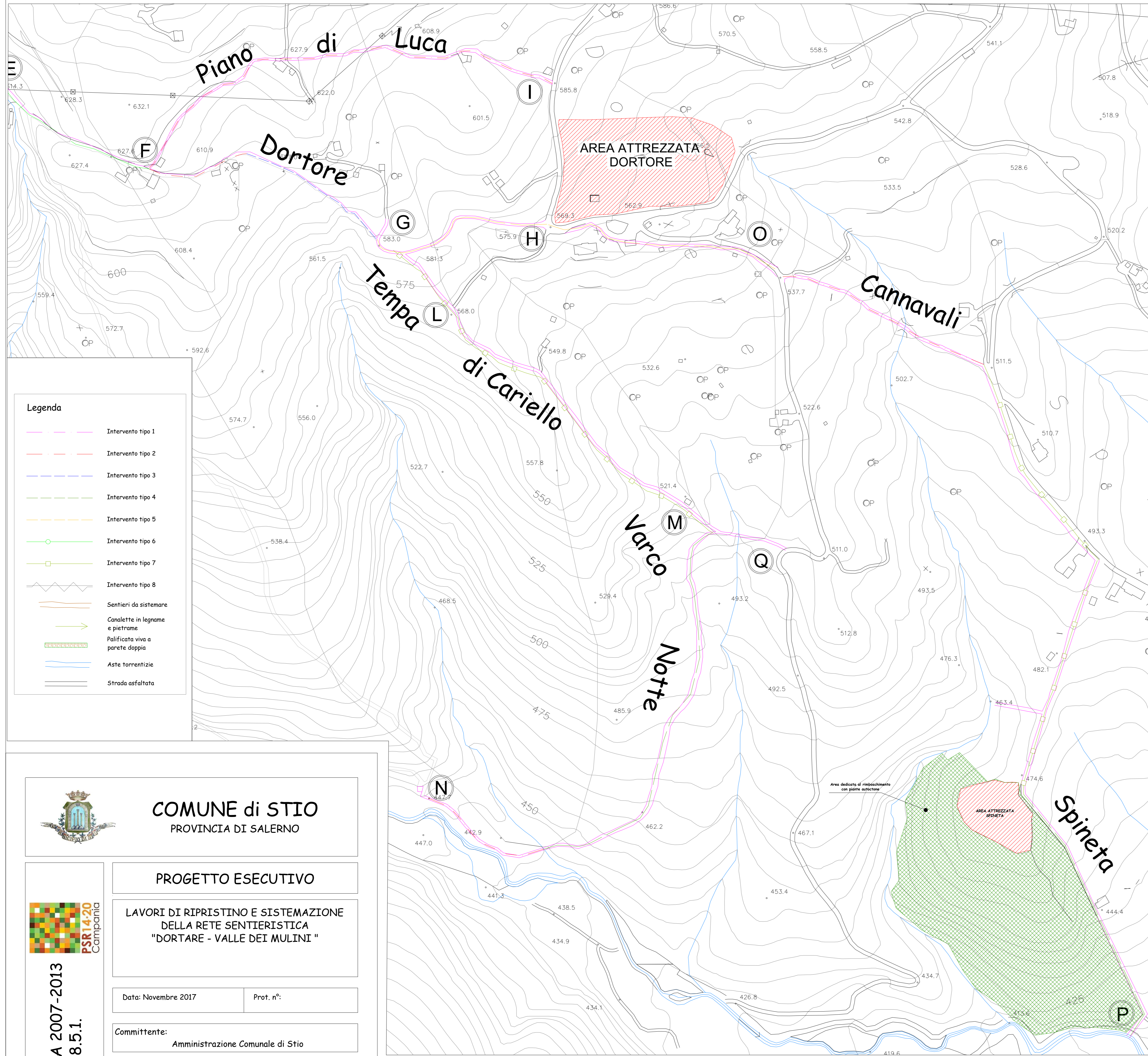
CARTA TECNICA REGIONALE CON UBICAZIONE DEGLI INTERVENTI - SCALA 1:2000
