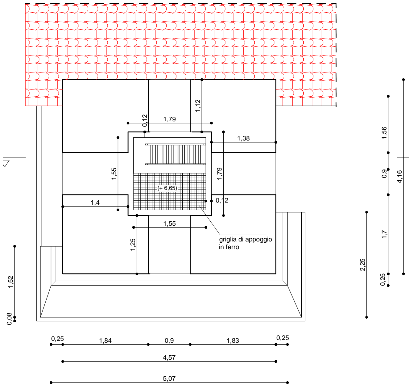
1° LIVELLO - Quota m. 6,65 scala 1:50
